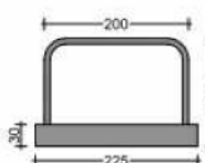
Listwa dwurzędowa Ø 8 mm
