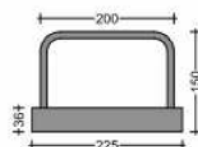
Listwa dwurzędowa Ø 10 mm
